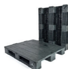
Ref. 1208 BP. 1200X1000 Carga estática:7000 Kg.
