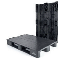
Ref. 1208 MPS 1200 x 800 | 1200 x 1000 Carga estática | Carga estática 4000 Kg | 4000 Kg
