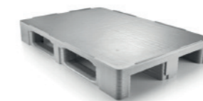
Ref. 1208 H. 1200X800 Carga estática:7500 Kg.
