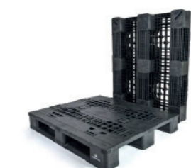
Ref. 1210 MP. 1200X1000 Carga estática:7000 Kg.
